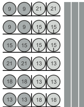
6 Sorten Tütenware, 12 Sorten Riegelware, 3 Schmalschächte* FS 1500 4/18 + 3
