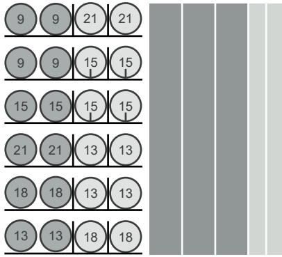
6 Sorten Tütenware, 12 Sorten Riegelware, 3 Normalschächte, 2 Schmalschächte* FS 2020 4/18 + 5
